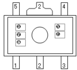
SOT-89-5
