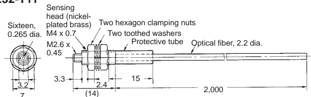
E32-T11
