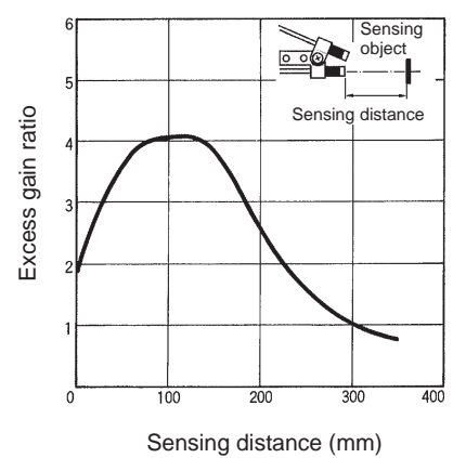
E32-T11L + E39-F3
