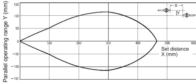
E32-T11L +E39-F1
