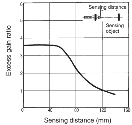
E32-D21L
