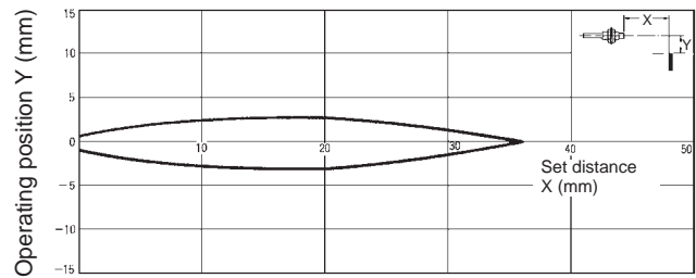
E32-D21L
