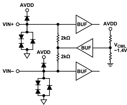
Figure 16. Analog Inputs ( V_{CM} \approx 1.4V )
