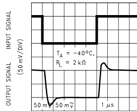
TIME (1 \mu s /DIV) DS011991-64
