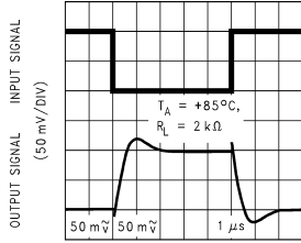
TIME (1 \mu s /DIV) DS011991-60
